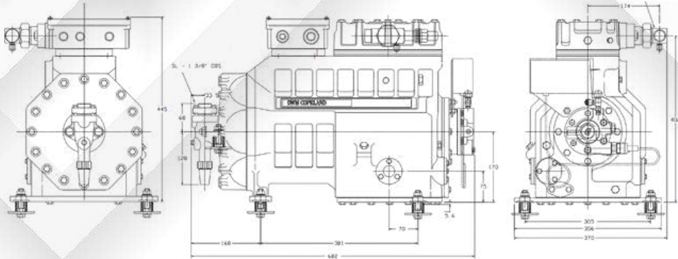
15 HP : Model: 4ML-15X
