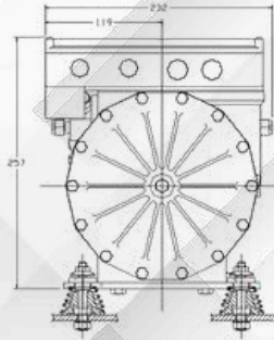
1.5HP : Model: KL-15X
