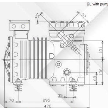
5 HP : Model: 2DC-50X
