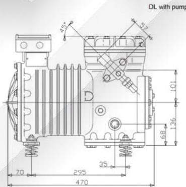
3 HP : Model: LF-30X
