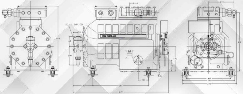
10 HP : Model: 3DS-150X
